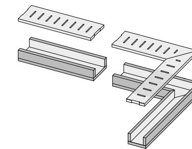
GRIGLIA 15 15x60 . 6"x24" 20 mm Nat. Ret. RII CANALINA 15x8x60 . 6"x3"x24" 20 mm Nat. Ret. RII
